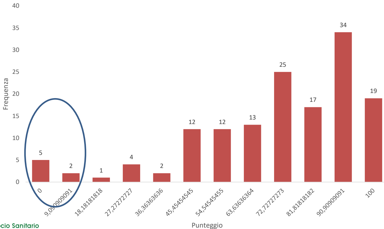
Resoconto Punteggi questionario di autovalutazione
